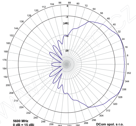
Vyzařovací diagram
