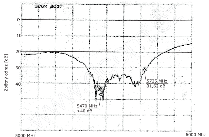
Graf přizpůsobení
